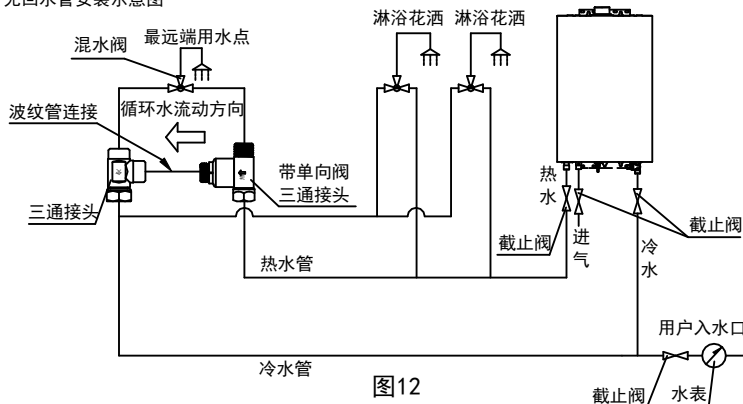
无回水管安装示意图
